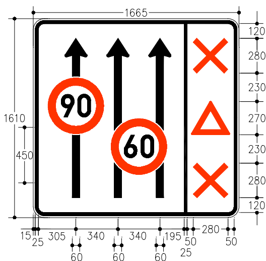
III-5α: 3ιχνος διατομή με λωρίδα έκτακτης ανάγκης
