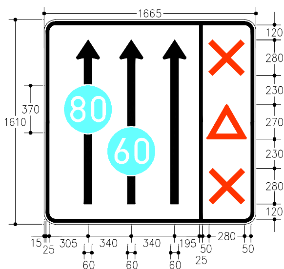
III-4α: 3ιχνος διατομή
