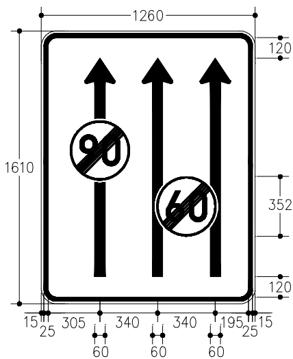
III-6α: 3ιχνος διατομή
