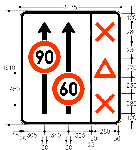
III-5β: 2ιχνος διατομή με λωρίδα έκτακτης ανάγκης
