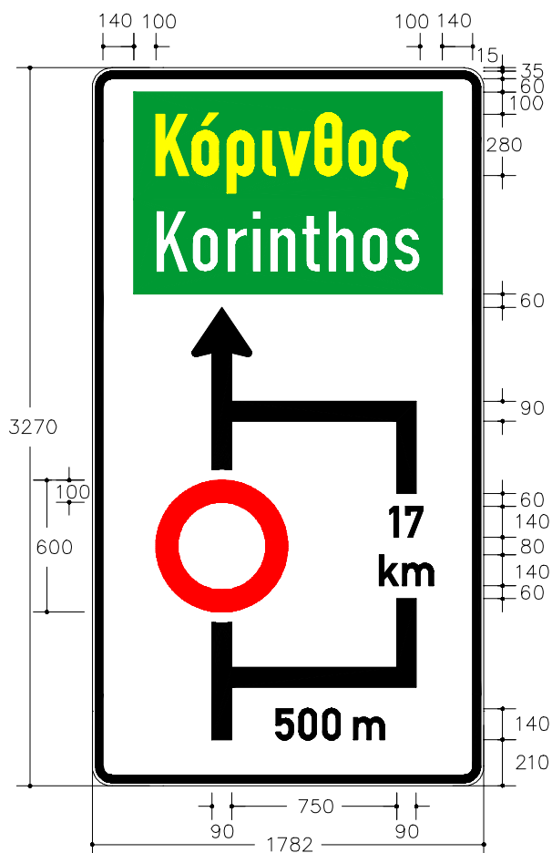
Σχήμα III-8: Υποχρεωτική παράκαμψη στα (π.χ. σε αυτοκινητόδρομο 500) m, μήκους (π.χ. 17) km για τον προορισμό (π.χ. Κόρινθος)
