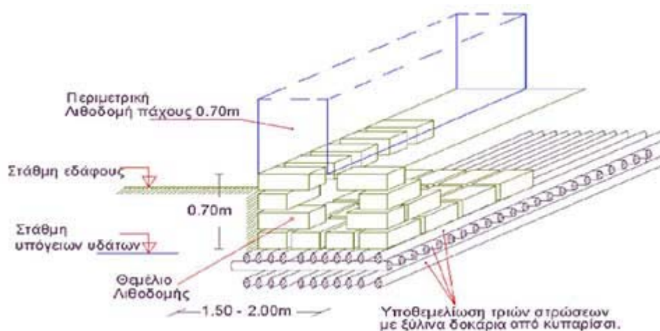
Εικ.: Τυπική θεμελίωση παραδοσιακών κτιρίων στην πόλη της Λευκάδας.
