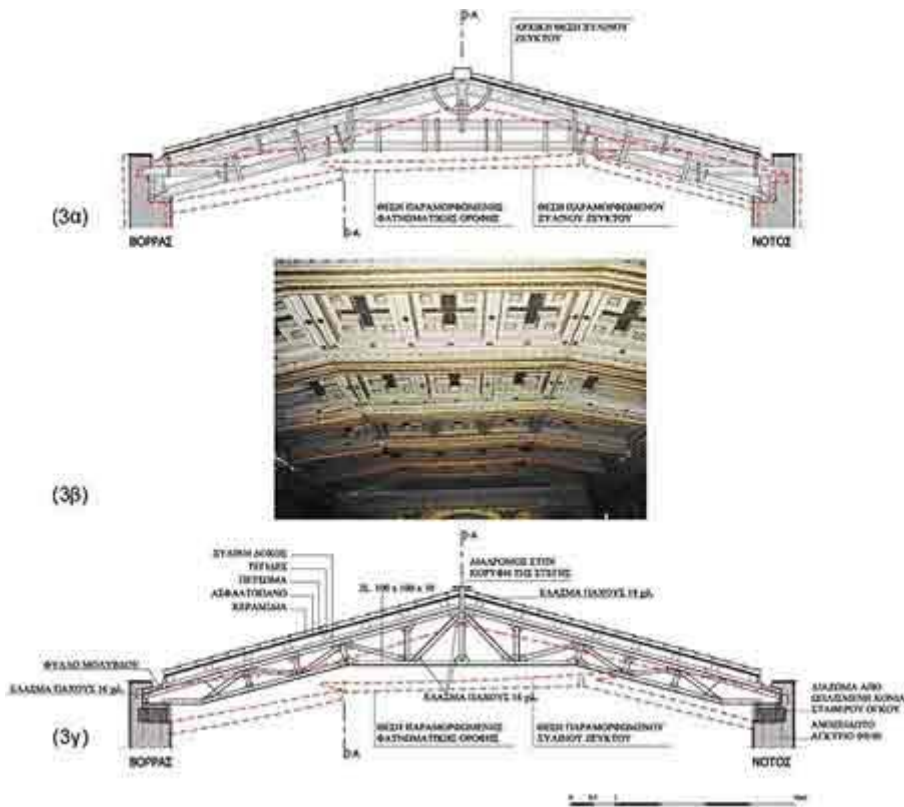
Εικ.: Σχέδιο υπάρχοντος ξύλινου ζευκτού (3α) και νέου μεταλλικού ζευκτού (3γ). Άποψη της ανηρτημένης από αυτά φαντωματικής οροφής (3β).
