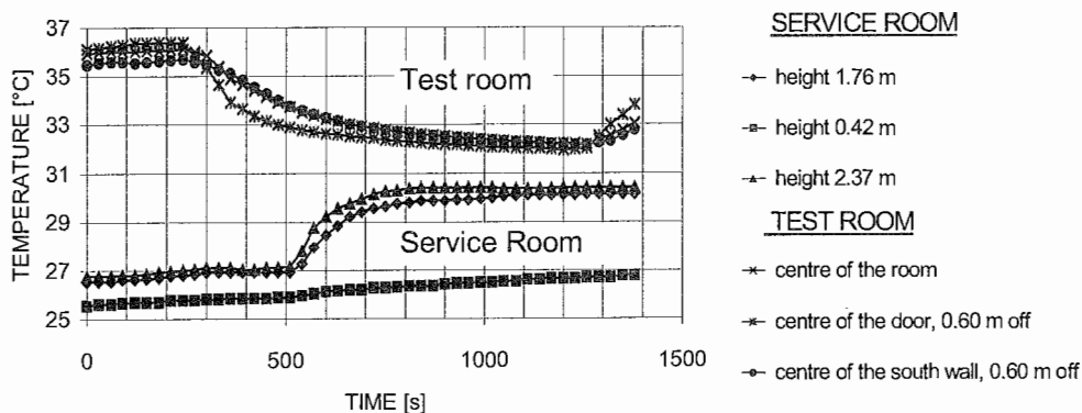
Σχήμα 2: Μεταβολή της θερμοκρασίας του αέρα με το χρόνο κατά την αποκατάσταση επικοινωνίας δια μέσου ενός μεγάλου ανοίγματος μεταξύ δύο θαλάμων.
