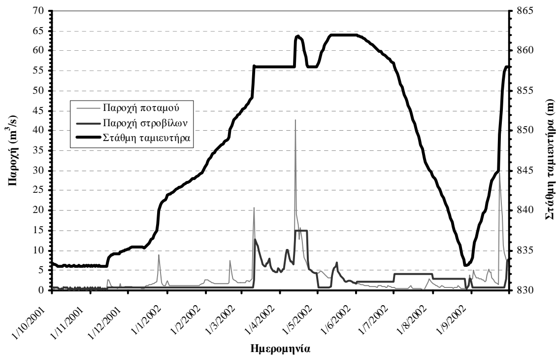
Γράφημα 7: Λειτουργία ταμιευτήρα για το πλέον ξηρό έτος – Μέγιστη παροχή στροβίλων Q_{max}^t = 14 \text{ m}^3/\text{s}
