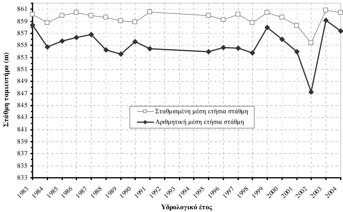
Γράφημα 6: Αριθμητική & σταθμισμένη μέση ετήσια στάθμη ταμιευτήρα
