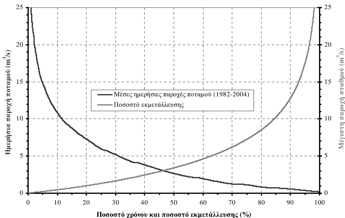
Γράφημα 2: Μένες ημερήσιες παροχές π. Αλιάκμονα και ποσοστό εκμετάλλευσης για παραγωγή ενέργειας
