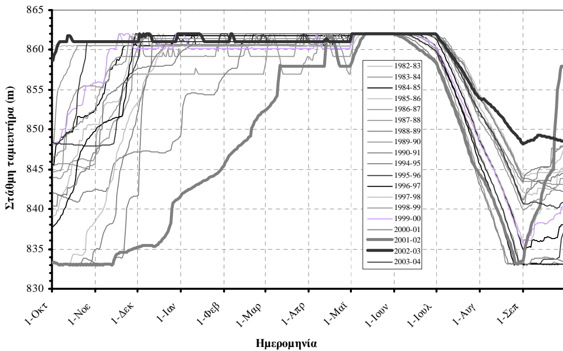
Γράφημα 5: Λειτουργία ταμιευτήρα – ημερήσια μεταβολή στάθμης
