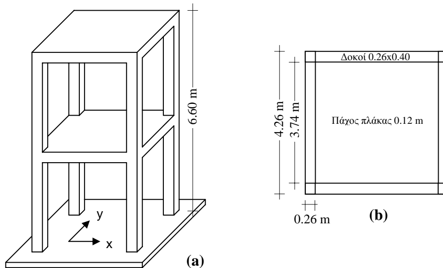
Σχήμα 1. Αξονομετρικό (1α) και κάτοψη κτηρίου (1β)
