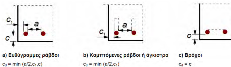
Σχήμα 8.3 : Τιμές του c_d για δοκούς και πλάκες
