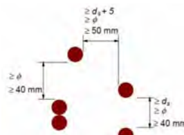
Σχήμα 8.15 Σωλήνες
