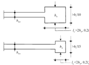
Σχήμα 5.10 Ελάχιστο πάχος περισφισμένων στοιχείων άκρων
