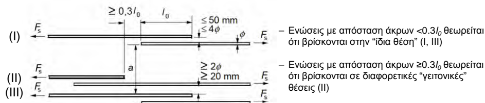
Σχήμα 8.7 : Ενώσεις με υπερκάλυψη
