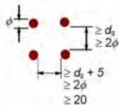
Σχήμα 8.14 Τένοντες
