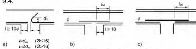
Σχήμα 9.4: Αγκυρώσεις σε ενδιάμεσες στηρίξεις
