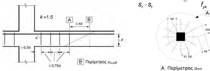
Σχήματα 9.10α, 6.22 Διάταξη συνδετήρων έναντι διάτρησης
