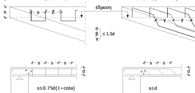
Συνδετήρες
