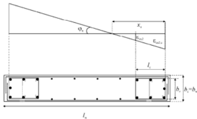
Σχήμα 5.8 Περισιφισμένο ελεύθερο άκρο τοιχώματος
