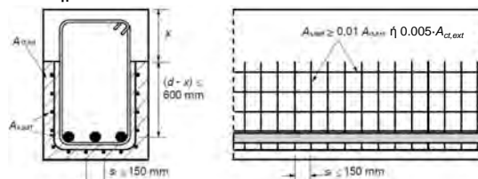
Σχήμα J.1 Διάταξη επιφανειακού οπλισμού
