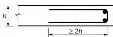
Σχήμα 9.8 : Οπλισμός ελεύθερου άκρου πλάκας
