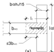
Σχήμα 5.11 Τοίχωμα ΚΠΥ με εγκάρσιο πέλμα
