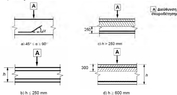
Σχήμα 8.2 Διάκριση συνθηκών συνάφειας
