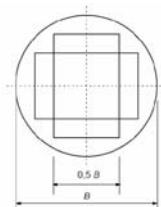
Σχήμα 9.12 Κυκλικό πέδιλο
