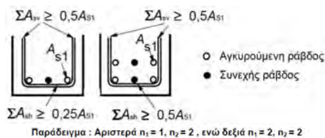
Σχήμα 8.11 Επιπρόσθετος οπλισμός στη ζώνη αγκύρωσης ράβδων μεγάλης διαμέτρου όπου δεν υπάρχει θλίψη στην εγκάρσια διεύθυνση
