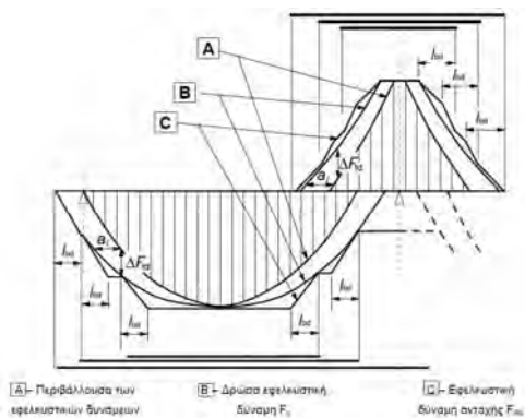
Σχήμα 9.2 Κλιμάκωση του διαμήκου εφελκόμενου οπλισμού δοκών
