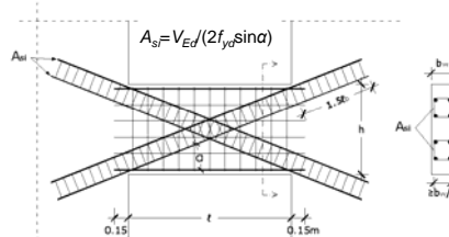
Σχήμα 5.12 Δοκός σύζευξης με διαγώνιο οπλισμό
