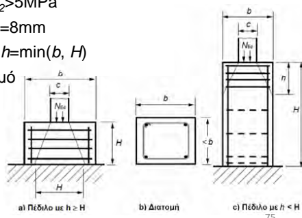
Σχήμα 9.14 Οπλισμός εγκάρσιας διάρρηξης πεδύλου επί βράχου
