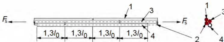
Σχήμα 8.13 Διάταξη διαδοχικής ένωσης με υπερκάλυψη δέσμης τριών ράβδων υπό εφελκυσμό που περιλαμβάνει τέταρτη πρόσθετη ράβδο μόνο στο συνολικό μήκος υπερκάλυψης 4(1.3l_0) = 5.2l_0
