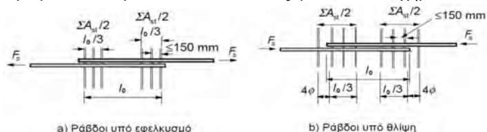
Σχήμα 8.9 Διάταξη εγκάρσιων οπλισμών στο μήκος υπερκάλυψης
