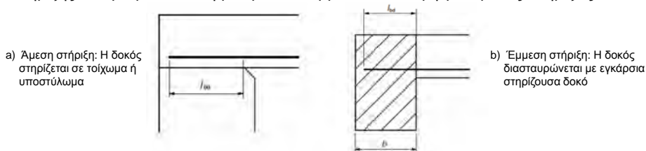
Σχήμα 9.3 Αγκύρωση των κάτω ράβδων σε ακραίες στηρίξεις
