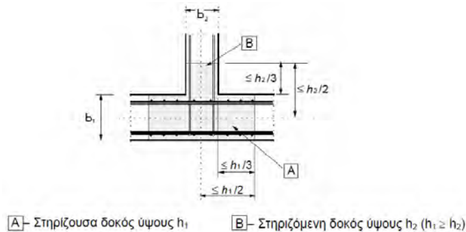
Σχήμα 9.7 Τοποθέτηση οπλισμού ανάρτησης (κάτοψη)
