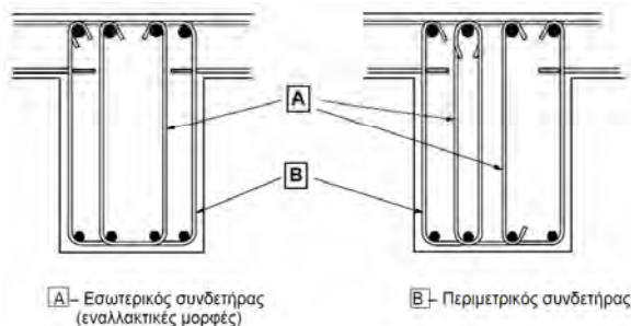
Σχήμα 9.5 : Παραδείγματα οπλισμών διάτμησης
