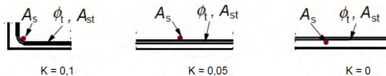
Σχήμα 8.4 : Τιμές του K για δοκούς και πλάκες
