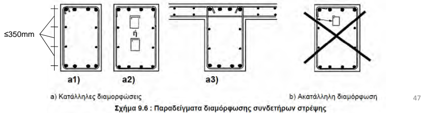
Σχήμα 9.6 : Παραδείγματα διαμόρφωσης συνδετήρων στρέψης
