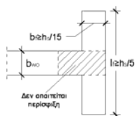
Σχήμα 5.9 Τοίχωμα ΚΠΜ με επαρκές εγκάρσιο πέλμα
