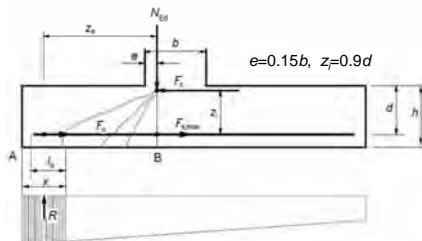
Σχήμα 9.13 Υπολογισμός και αγκύρωση κύριου οπλισμού
