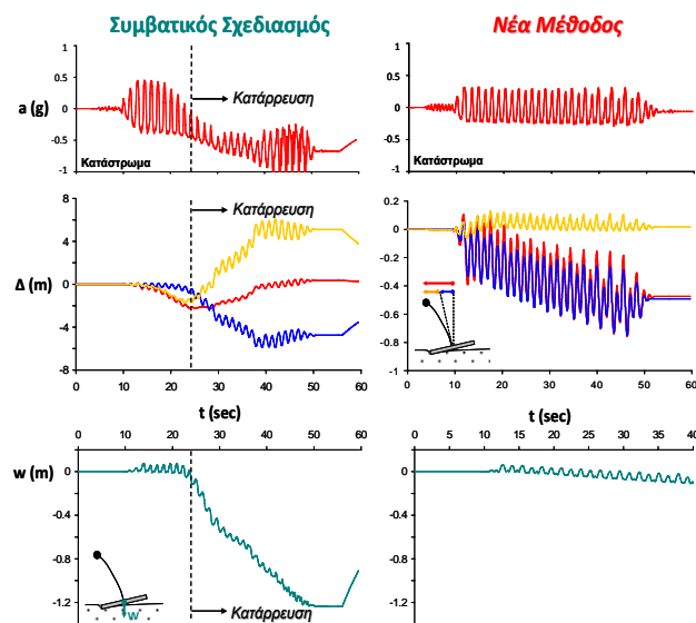
Σχήμα 6. Σύγκριση των δύο συστημάτων για σεισμική διέγερση που υπερβαίνει τον σχεδιασμό (ημιτονική διέγερση 30 κύκλων, 1 Hz, 0.4 g). Figure 6. Comparison of two systems for excitation beyond design limits (sinusoidal motion, 30 cycles, 1 Hz, 0.4 g).
