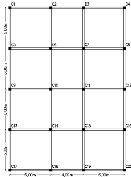
Σχ. 1 Κάτοψη κτιρίου
