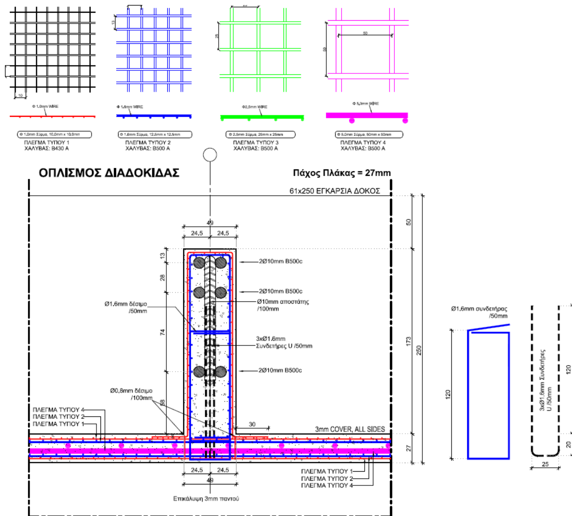
Σχ. 3 Διατομή T κάτω πέλματος
