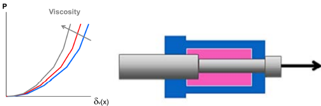
Σχ. 6 Ελατήρια υπό ελκυσμό, σιλικόνη πάντα σε σύνθλιψη, δύναμη συνάρτηση της μεταβολής του όγκου και του ιξώδους.
