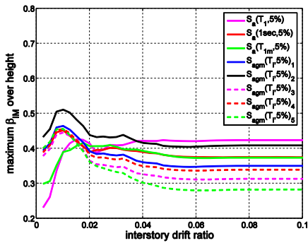
(a) maximum dispersion of IDR given IM (3ELF)
