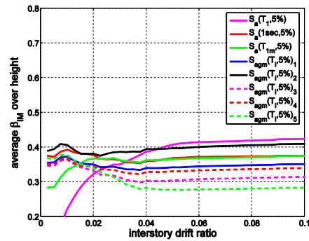
(b) average dispersion of IDR given IM (3ELF)
